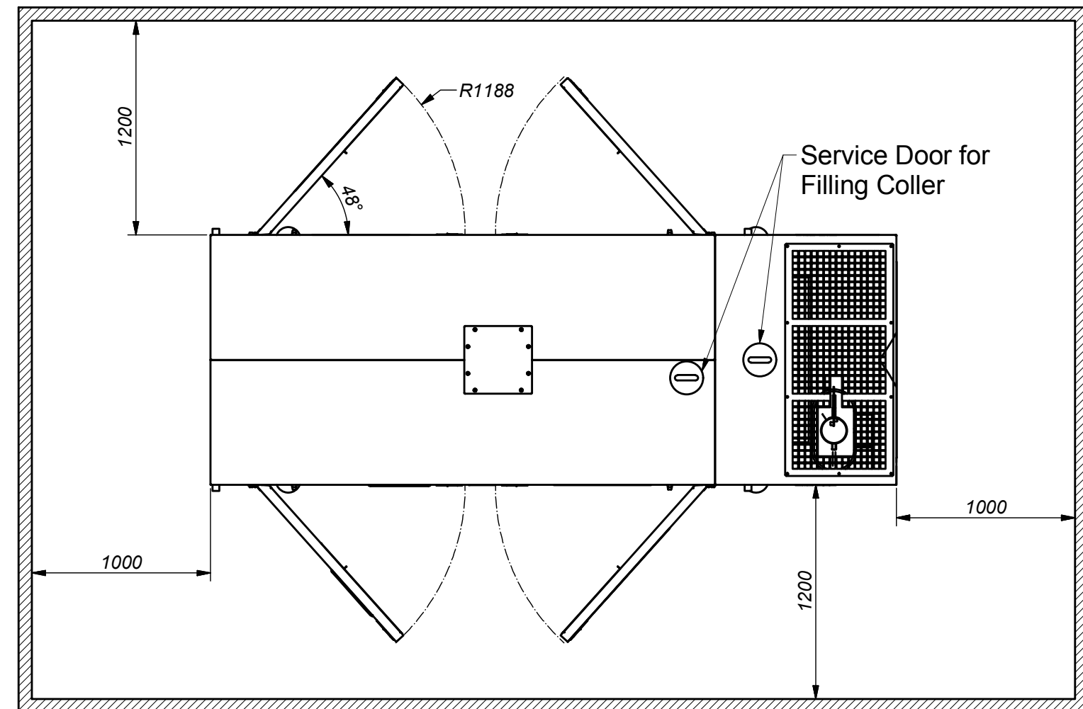
MAINTENANCE SPACE ( 1 : 30 )
